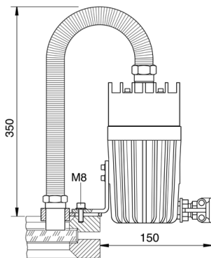
Befestigung der Lichtquelle auf Schauglasarmaturen nach oder ähnlich DIN 28120 / 28121 mit Winkel «W»
