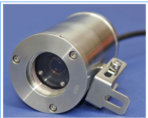
Explosionssgeschützte Videokamera VIDEOLUX in Edelstahl-Ausführung, Typ miniZoom, Ex d IIB (C), Ex II 2 G + D
