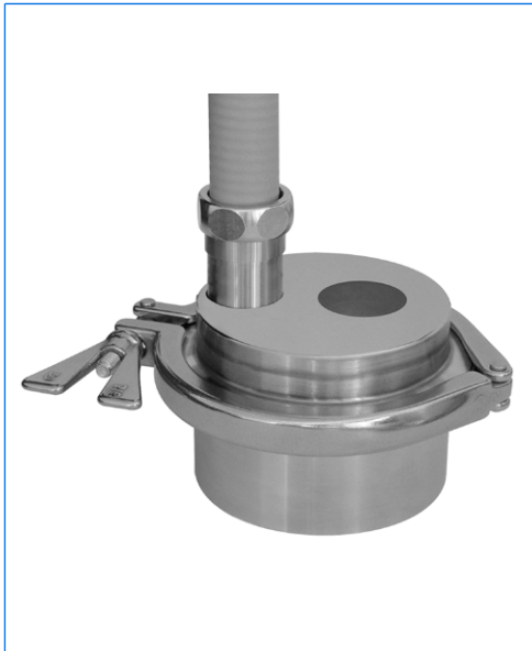
Metallverschmolzenes Schauglas, 4", mit eingestecktem Lichtleiter der fibroLUX-Fiberoptik-Schauglasleuchte
