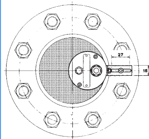
Befestigung «W»
