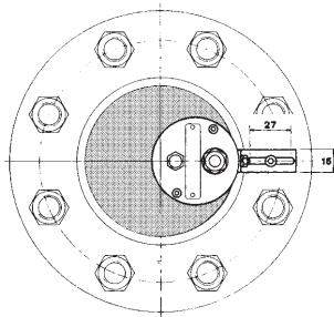
Befestigung «W»
