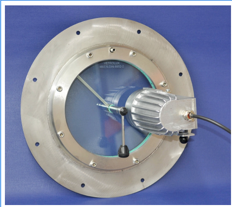
Oblò VETROLUX® simile a DIN 28120, PN 0, con flangia saldata per montaggio diretto sulla parete di un fermentatore, attrezzato di tergicristallo centrale, tipo W, lava vetro, tipo SVSN e di proiettore anti-deflagrante CHEMLUX®, tipo FHEL 50 dHV, 50 W, 230 V, Ex d II C T3, Ex II 2 G + D, con temporizzatore V incorporato
