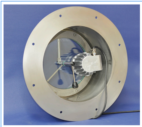
Oblò VETROLUX® sim. a DIN 28120, DN 200, PN 0, con flangia per fissaggio esterno contro la parete di un fermentatore in cemento armato, con tergiacristallo centrale, lava vetro e proiettore AD-PE CHEMLUX®, tipo FKEL 50 dH, 50 W, 24 V, Ex d II C T3, Ex II 2 G + D, fissaggio del proiettore con articolazione sferica
