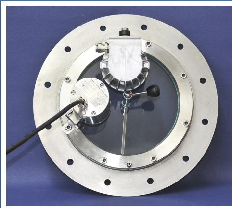
Oblò VETROLUX® simile a DIN 28120, PN 0, con flangia saldata per montaggio diretto sulla parete di un fermentatore, attrezzato di tergicristallo, lava vetro, proiettore AD-PE CHEMLUX® e sistema di videocamera AD-PE VIDEOLUX
