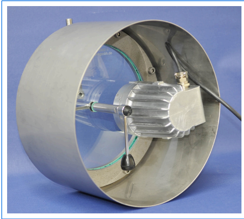
Oblò VETROLUX® sim. a DIN 28120, DN 200, PN 0, saldato su un tubo da sigillare nella parete di un fermentatore, con tergiacristallo centrale, lava vetro e proiettore AD-PE CHEMLUX®, tipo FKEL 50 dH, 50 W, 24 V, Ex d II C T3, Ex II 2 G + D, fissaggio del proiettore con articolazione sferica
