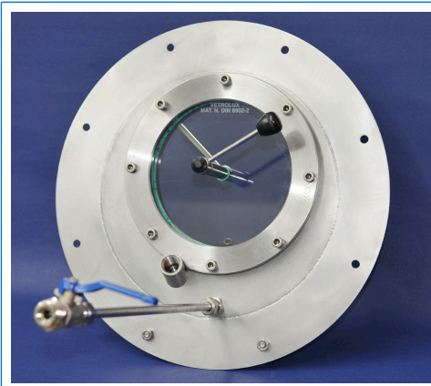
Oblò VETROLUX® simile a DIN 28120, PN 0, con flangia saldata per montaggio diretto sulla parete di un fermentatore, attrezzato di tergicristallo centrale, lava vetro e manicotto per montaggio segnalatore di schiuma
