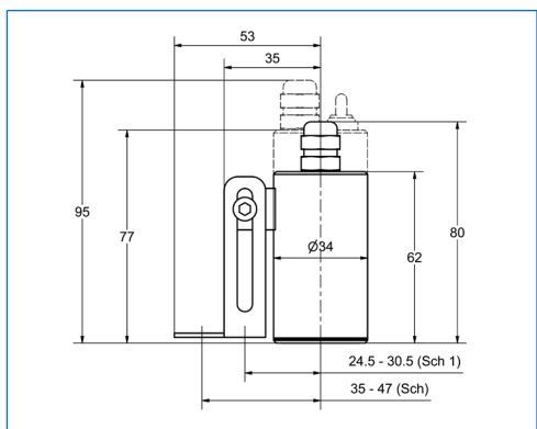
Micro-proiettore LED, tipo MVLR 2 LED, 2 W, 24 V AC/DC, con interruttore «marcia-arresto» «E» incorporato, montato su oblò avvitato VETROLUX similare a DIN 11851, DN 32, PN 6
